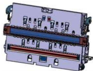
Верхняя часть блока детекции
